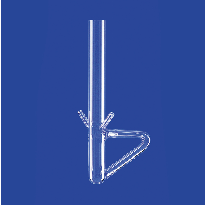
Schmelzpunktbestimmungsapparate nach Thiele
