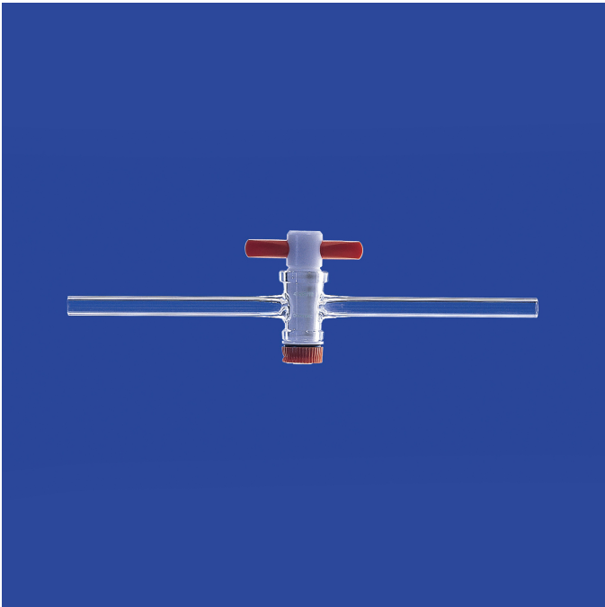
Einweg-Kegelhähne mit PTFE-Küken
